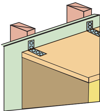
Ｌ字金具で下地材に固定する
