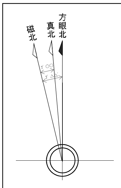
図：「方眼北」・「真北」・「磁北」の関係
